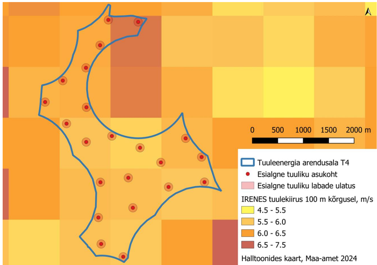
Joonis 10. Hinnanguline tuulekiirus tuuleenergia arendusosal T4 100 m kõrgusel maapinnast. Alus: Keskkonnaagentuur IRENES projekt.
