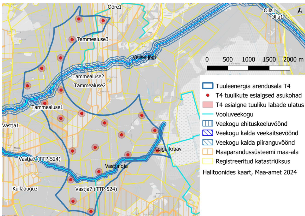
Joonis 4. Tuuleenergia arendusale T4 jäävad vooluveekogud ja nendega seotud kitsendused ning maaparandussüsteemi maa-alad.
