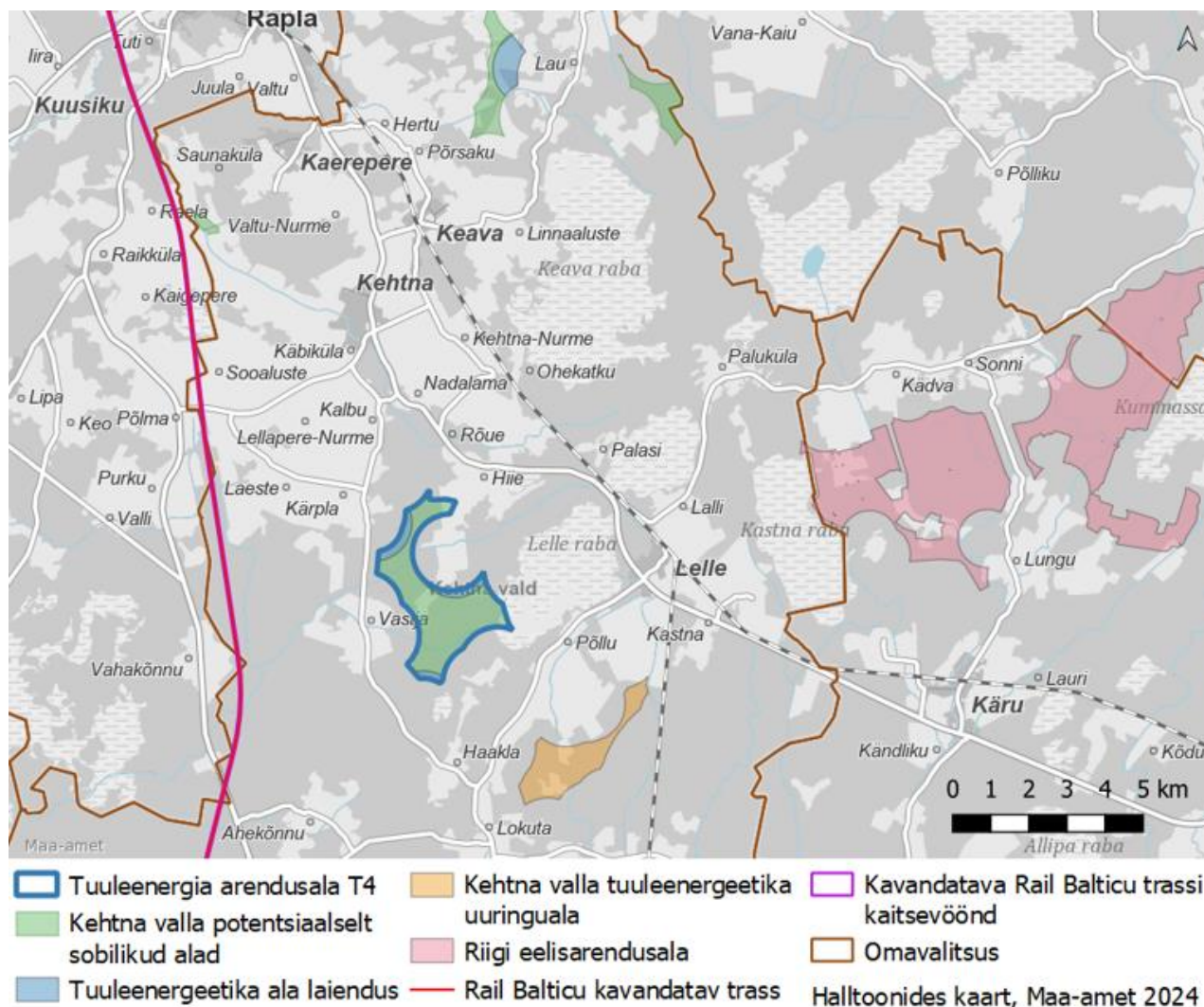
Joonis 12. Tuuleenergia arendusala T4 ning Kehtna vallas paiknevad teised potentsiaalselt sobilikud tuulealad ja nende laiendused, RB trass ning riigi eelisarendusala.
